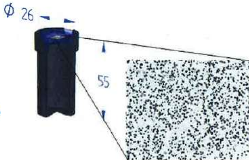
Abbildung 1: Kernspurdetektor (mit Vergrößerung des Polymer-Chip mit Spuren des Alpha-Zerfalls), Abmessungen in mm
